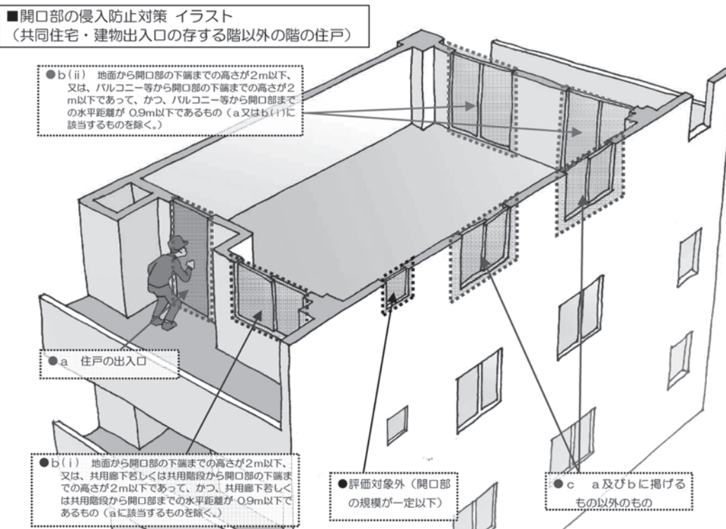
図2 建物の出入口の存する階以外の階の住戸の開口部
