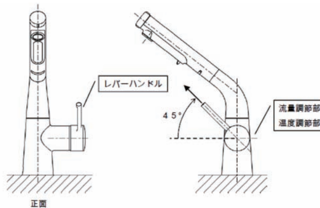
図9 水優先吐水機構—台所水栓（レバーハンドルが水栓胴の左右側面に位置する場合）の例
