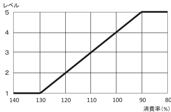
図 1 LR HU 1.1.1 の評価レベルと消費率の関係
