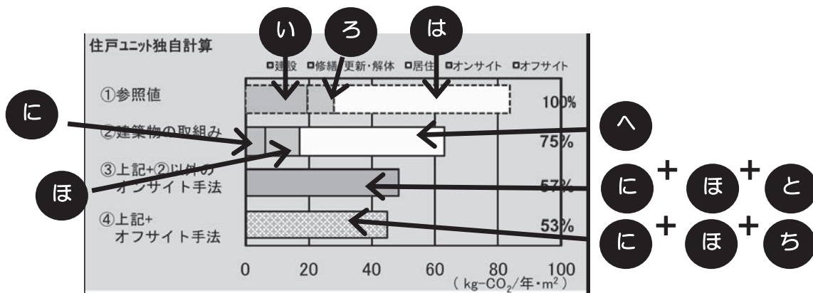
図 2.16 「住戸ユニット独自計算」の「ライフサイクル CO 2 （温暖化影響チャート）」の例（一部）
