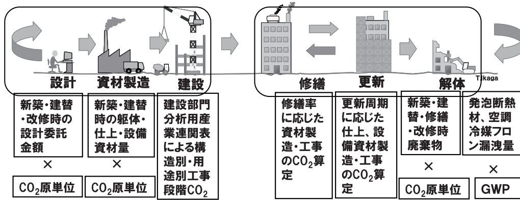
図 3.9 建物の LCA 指針における CO 2 排出量の積上げ（「建設」「修繕・更新・解体」時）
