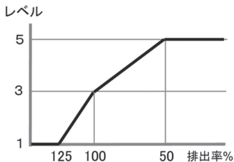
図 LR HU3.1.1 の評価レベルと排出率の関係
