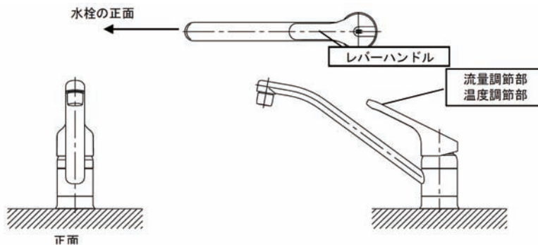
図 7 水優先吐水機構—台所水栓（正面で湯が吐出しない構造）の例
