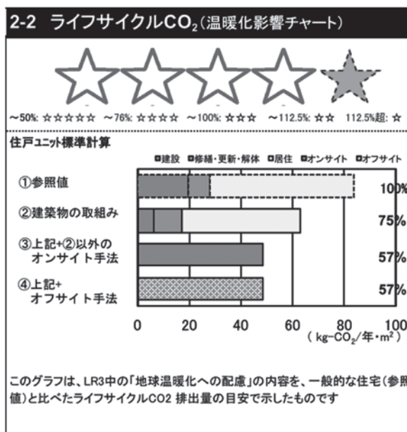
図 2.19 「2-2 ライフサイクル CO_2 (温暖化影響チャート)」の表示例
