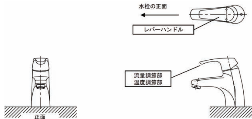
図10 水優先吐水機構—洗面水栓の例
