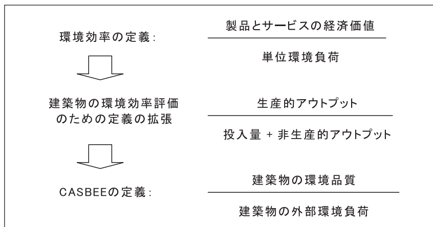
図 3.2 環境効率（エコ・エフィシエンシー）の概念からBEEへの展開
