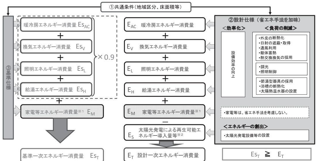
図 4 H25 省エネ基準における一次エネルギー消費量基準の評価方法
