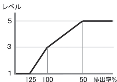
図 3.10 LR_{HU}3.1.1 の評価レベルと排出率の関係
