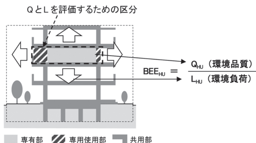
図 3.3 CASBEE-住戸ユニット（新築）における「QとLを評価するための区分」
