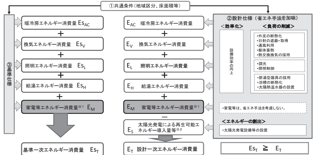
図 4 H25 省エネ基準における一次エネルギー消費量基準の評価方法
