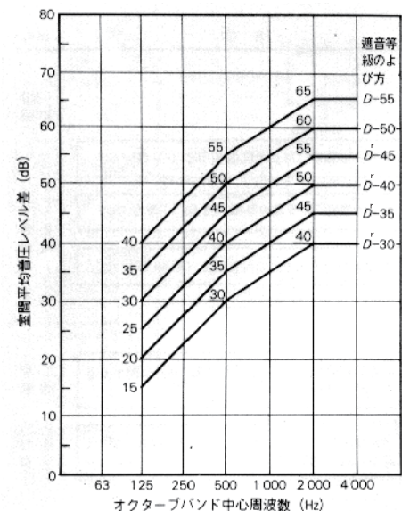
■参考）空気音遮断性能の周波数特性と等級（等級曲線）（JIS A 1419-1）
