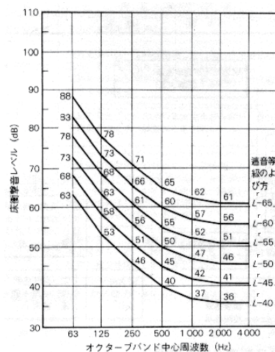
■参考）床衝撃音遮断性能の周波数特性と等級（等級曲線）（JIS A 1419-2）
